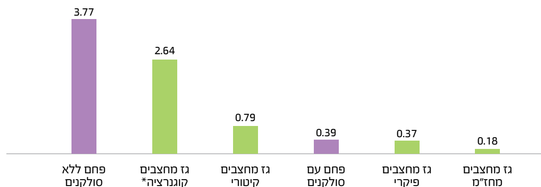
איור 6 פליטה סגולית לאוויר של חלקיקים מסוגי יחידות חשמל שונות, גרם חלקיקים/קוט"ש
